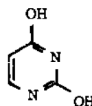
uracil
